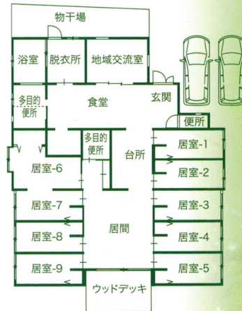
■間取り
